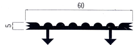
消音用ゴム詳細図
