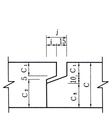
継手詳細図
